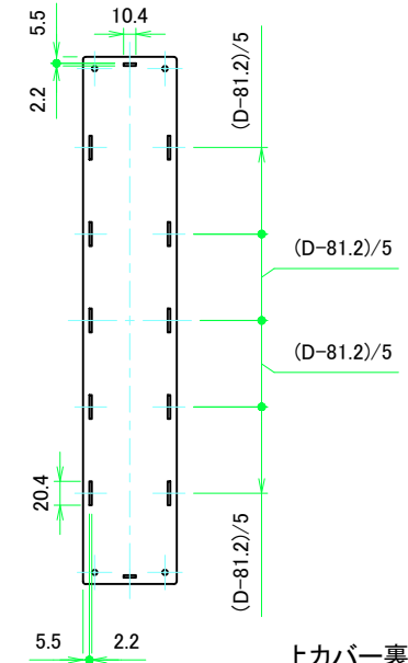
上カバー裏面 / Top cover Backside
